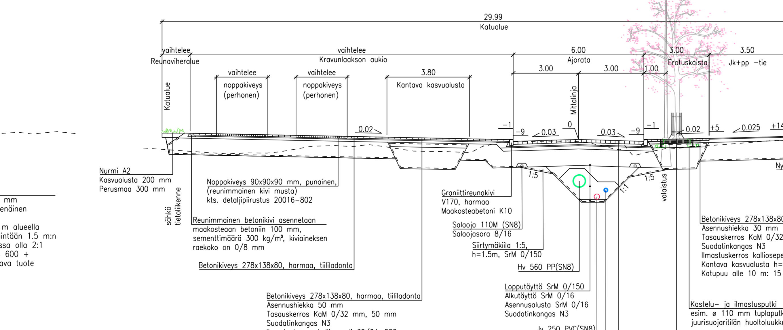
KITTELÄNTIE (PL 520) TYYPPIPOIKKILEIKKAUS 1:100
