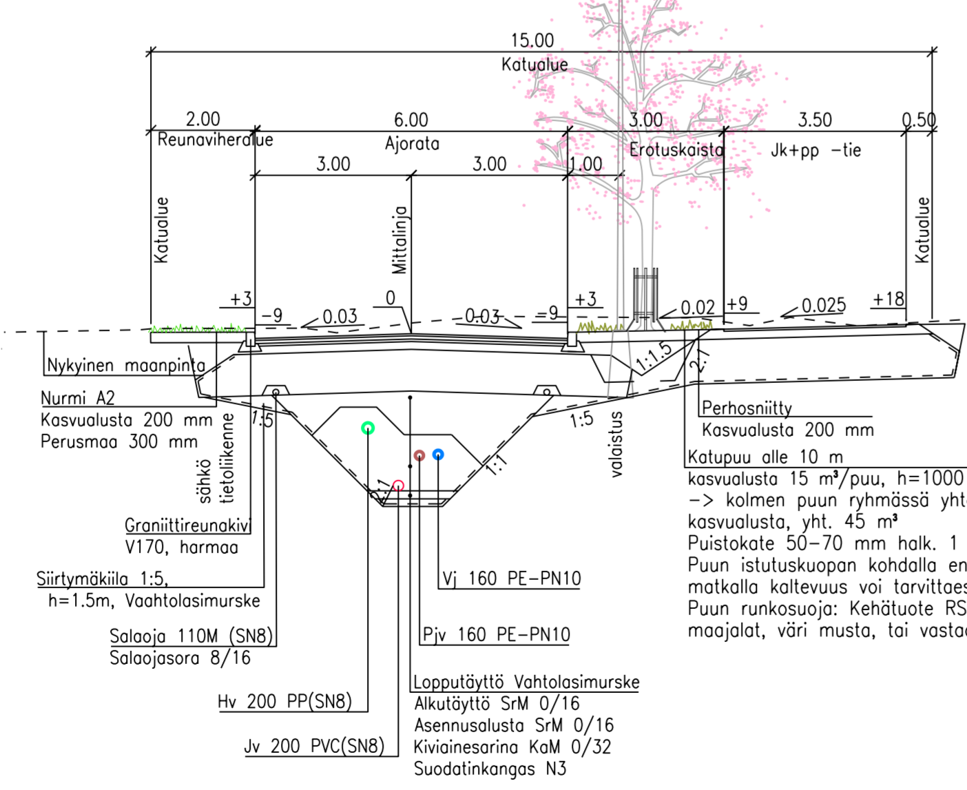
KITTELÄNTIE (PL 250) TYYPPIPOIKKILEIKKAUS 1:100
