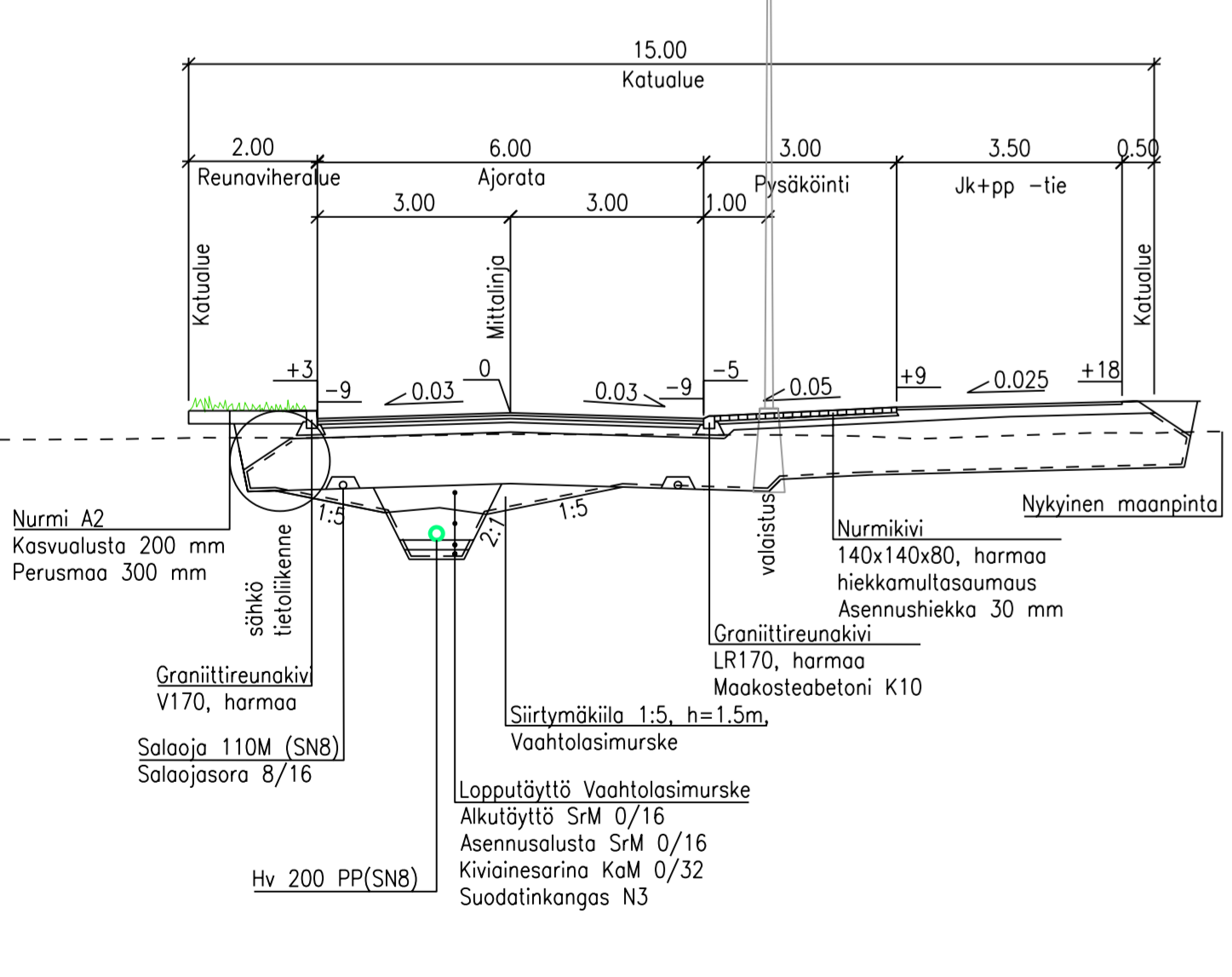
KITTELÄNTIE (PL 40) TYYPPIPOIKKILEIKKAUS 1:100
